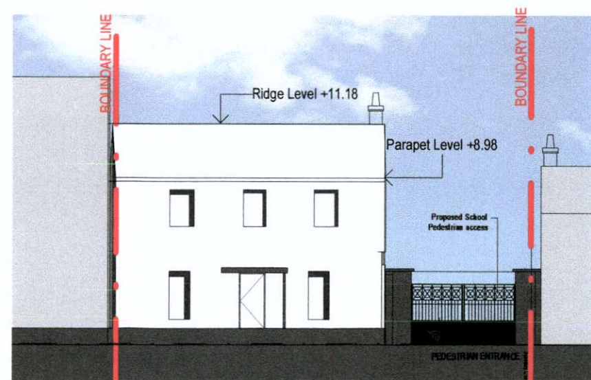
② Elevation BB 1 : 200
