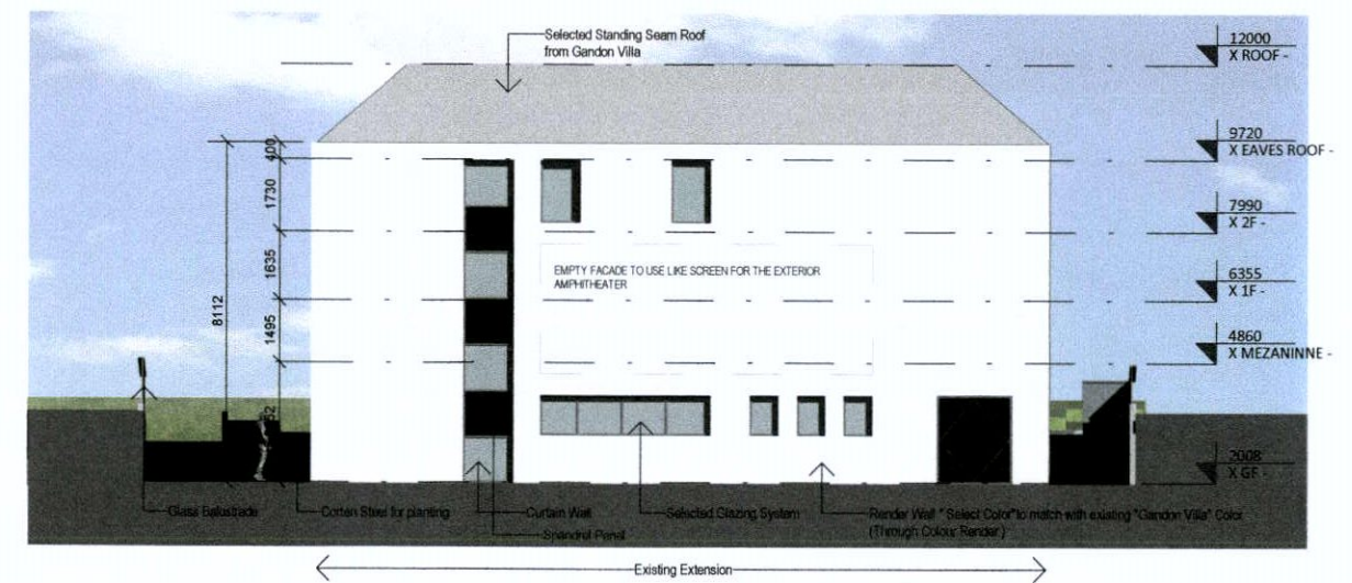
1 Elevation AA 1 : 200
