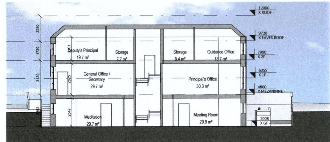
3 Section 03 1 : 200
